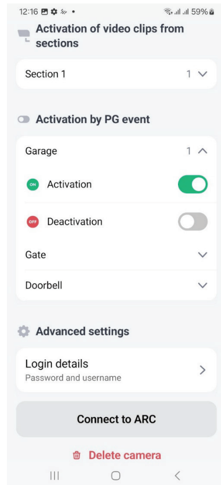
Obr. 8: aktivácia videoklipov
