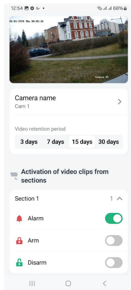
Obr. 5: Nastavenia toku
