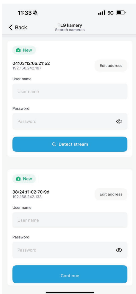
Obr. 3: Detekcia toku
