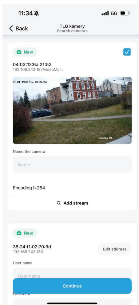
Obr. 4: náhľad prúdu
