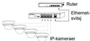
Fig. 2: Tilkoblingsskjema for Ethernet-svitsj
