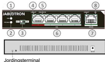
Fig. 1: Beskrivelse av produktets indre og ytre deler
