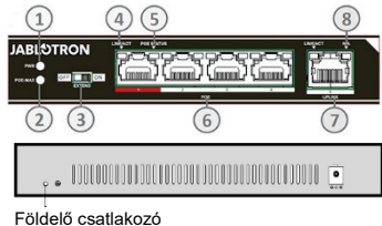
1. tápellátás kijelzője 2. PoE tápegység mutató 3. EXTEND kapcsoló a PoE tápegységet a növelje a maximális LAN kábelhossz 4. LAN eszköz aktivitás jelző 5. PoE tápegység használatának jelzője 6. RJ-45 csatlakozó a routerhez kapcsolat 7. RJ-45 csatlakozó a routerhez kapcsolat 8. LED nincs funkció
