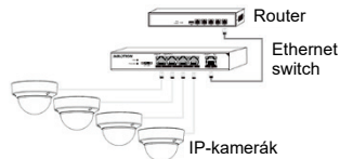
2. ábra: Ethernet switch csatlakozási diagram
