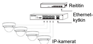
Kuva 2: Ethernet-kytkimen kytkentäkaavio
