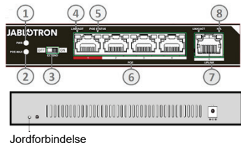
Fig. 1: Beskrivelse af produktets indre og ydre dele
