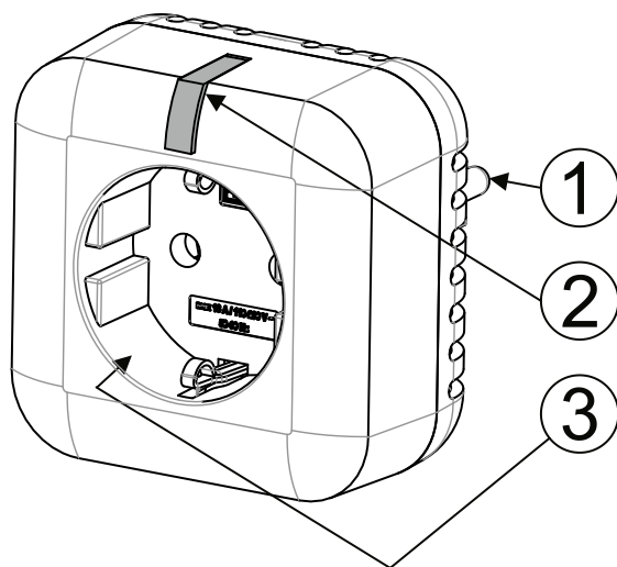
Fig. 1: Descrizione delle parti esterne del prodotto 1 – Spina UniSchuko; 2 – Pulsante funzionale / indicatore LED; 3 – Presa Schuko
