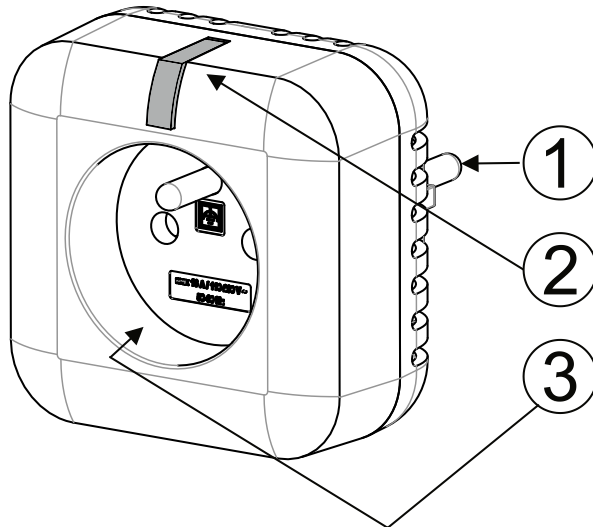
Fig. 1: Beskrivelse av de eksterne delene av produktet 1 - UniSchuko-plugg; 2 - funksjonsknapp / LED; 3 - fransk stikkontakt
