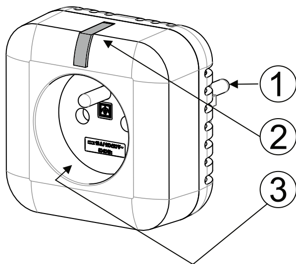
Fig. 1: Beskrivelse af produktets eksterne dele 1 - UniSchuko-stik; 2 - funktionsknap / LED; 3 - fransk stikkontakt
