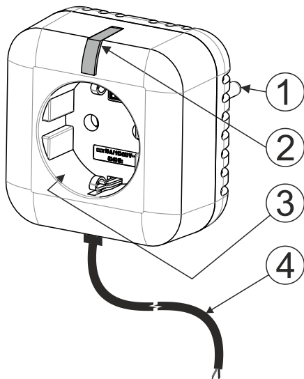
Bild 1: 1 – UniSchuko-kontakt, 2 – funktionsknapp/indikator; 3 – uttag, 4 – potentialfri kopplad utgångskabel Installation
