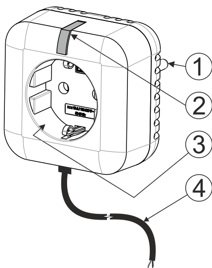
Rys. 1: 1 – wtyczka UniSchuko; 2 – przycisk funkcyjny/wskaźnik; 3 – gniazdo Schuko, 4 – bezpotencjałowy kabel wyjściowy
