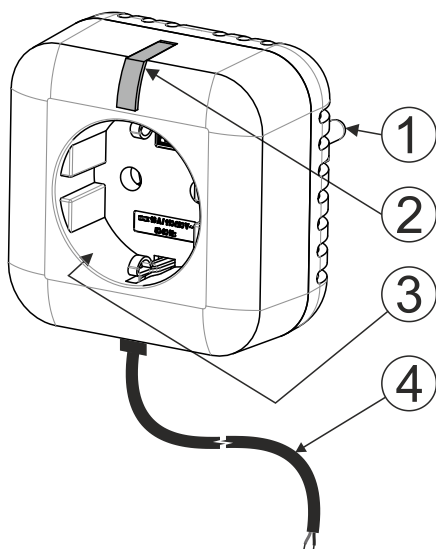
1. ábra: 1 – Schuko csatlakozó dugó; 2 – Funkció nyomógomb/LED visszajelző; 3 – Schuko csatlakozó aljzat, 4 – Potenciál mentes kapcsolt kimenet vezetéke
