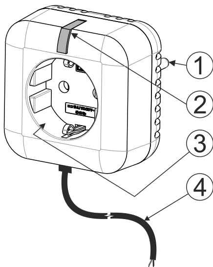
Fig. 1 : 1 – fiche UniSchuko ; 2 – bouton/indicateur de fonction ; 3 – prise Schuko, 4 – câble de sortie commuté sans potentiel
