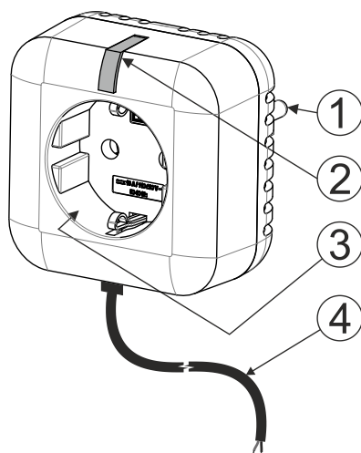
Obr. 1: 1 – vidlice typu UniSchuko; 2 – funkční tlačítko/LED; 3 – zásuvka typu Schuko, 4 – kabel spínaného bezpotenciálového výstupu
