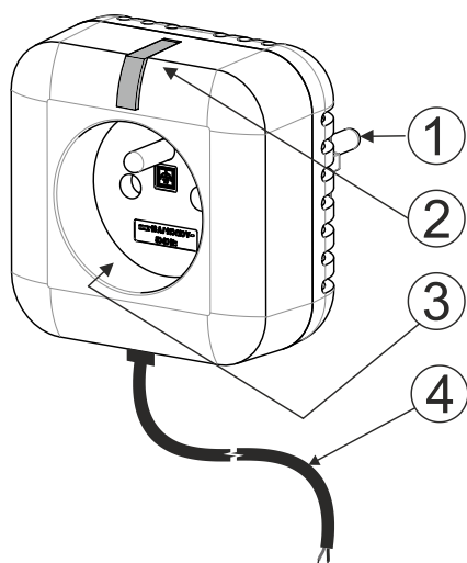
Rys.1: 1 – wtyczka UniSchuko; 2 – przycisk funkcyjny/wskaźnik; 3 – gniazdo French; 4 – bezpotencjałowy kabel wyjściowy
