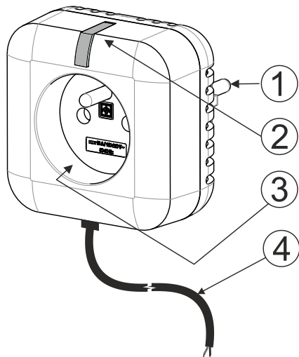
1. ábra: 1 – Schuko csatlakozó dugó; 2 – Funkció nyomógomb/LED visszajelző; 3 – csatlakozó aljzat French, 4 – Potenciál mentes kapcsolt kimenet vezetéke
