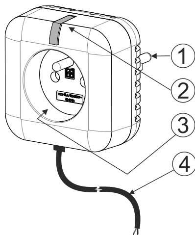
Obr. 1: 1 – vidlice typu UniSchuko; 2 – funkční tlačítko / LED; 3 – zásuvka typu French, 4 – kabel spínaného bezpotenciálového výstupu
