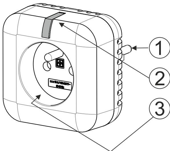
Obr. 1: 1 – vidlice typu UniSchuko; 2 – funkční tlačítko/LED; 3 – zásuvka typu French
