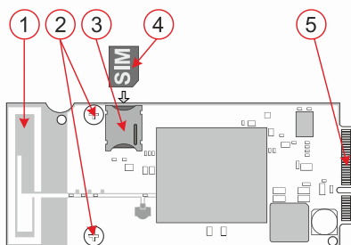
Obr. 1: Komunikátor JA-193Y-LITE
