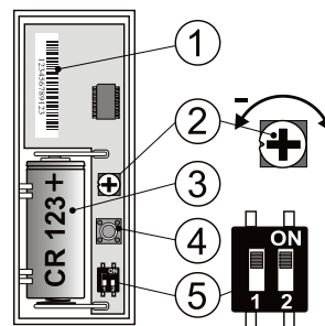
3. ábra: 1 – gyári sorozatszám; 2 – forgatható érzékenység szabályozó; 3 – CR-123 elem; 4 – szabotázs kontaktus; 5 – beállító kapcsoló.
