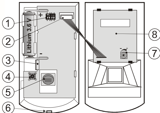
Obr. 1. DIP prepínače pre nastavenie vlastností detektora; 2. konektor; 3. západka; 4. sabotážny (Tammer) kontakt krytu; 5. PIR senzor; 6. západka krytu; 7. nastavenie citlivosti MW; 8. mikrovlnný detektor
