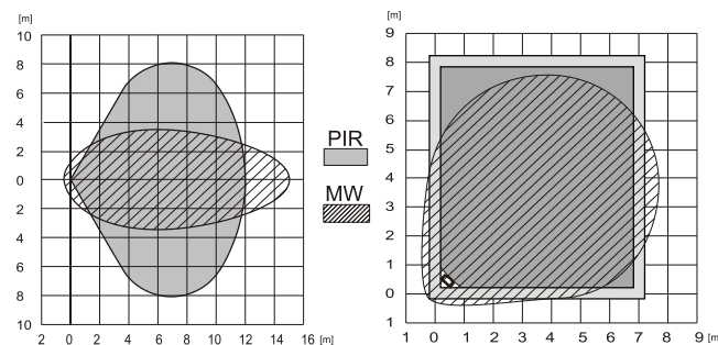
Obr. 2: detekčná charakteristika pokrytia vo voľnom priestore a v modelovej miestnosti – inštalácia v rohu.
