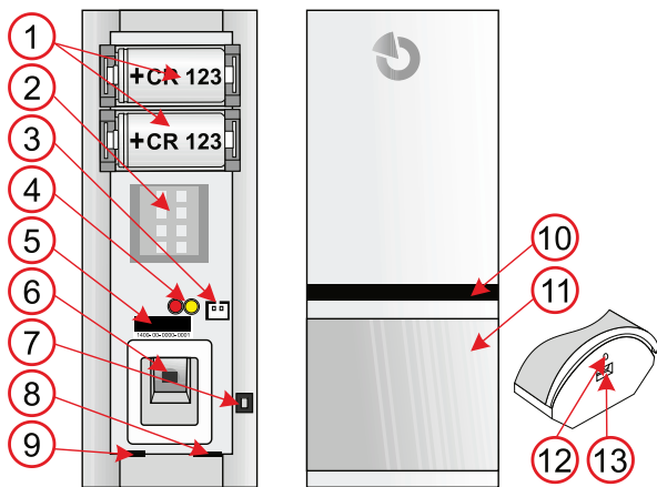
Obrázek 1: 1 – pouzdra pro baterie; 2 – MW senzor; 3 – konektor pro připojení sabotážního spínače kloubového držáku JA-191PL; 4 – LED pro indikaci stavů; 5 – sériové číslo; 6 – PIR senzor; 7 – sabotážní spínač; 8 – anténa; 9 – západka elektroniky; 10 – světlovod; 11 – čůčka PIR detektoru; 12 – otvor pro aretační šroub; 13 – západka krytu
