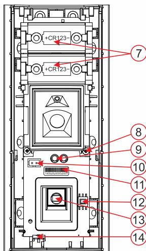
Obrázek: 7 – baterie; 8 – aretační šroubek modulu kamery; 9 – indikační LED; 10 – konektor externího sabotážního kontaktu; 11 – sériové číslo; 12 – sabotážní spínač; 13 – PIR senzor; 14 – západka DPS
