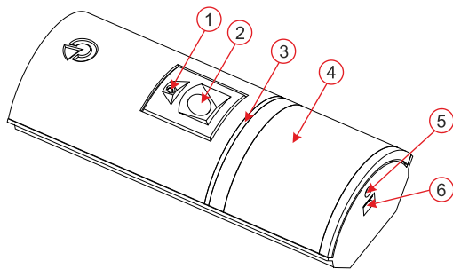
Obrázek: 1 – blesk pro přisvětlení; 2 – objektiv kamery; 3 – světlovod LED indikátorů; 4 – čočka PIR detektoru; 5 – aretační šroubek; 6 – západka krytu
