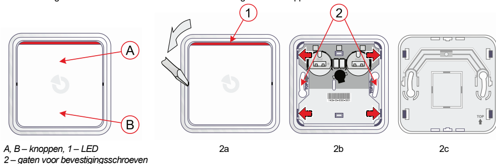
Fig. 1: Beschrijving van externe onderdelen van het product en indeling van de knop in 3 delen
