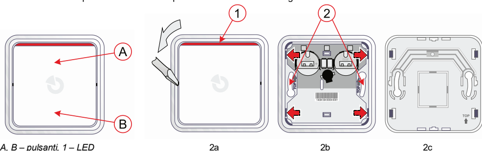
A, B – pulsanti, 1 – LED 2 – fori per le viti di fissaggio
