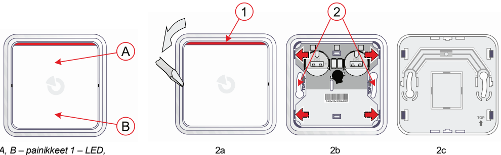
A, B – painikkeet 1 – LED, 2 – reiät kiinnitysruuveja varten
