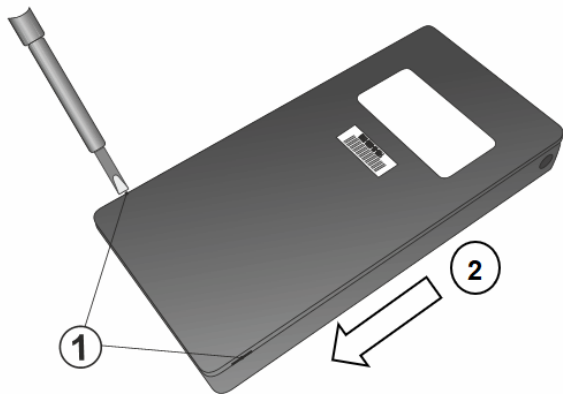
Obr. 4: Spôsob otvorenia tiesňového tlačidla: 1. priestor pre zapáčenie na otvorenie vrchného krytu (pomocou plochého skrutkovača na oboch stranách tlačidla). 2. Smer otvorenia (po zapáčení kryt vysunúť smerom dohora).
