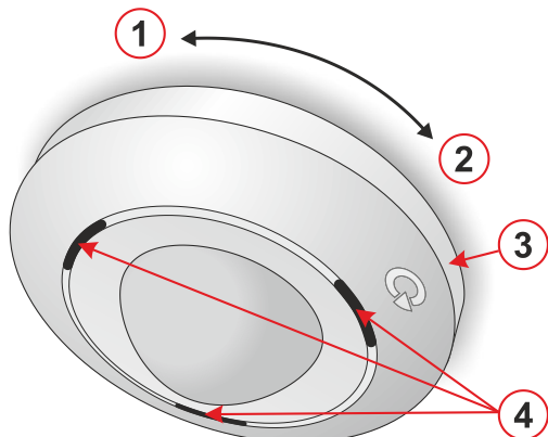
Obrázek 1.: 1 – směr pro uvolnění detektoru; 2 – směr pro upevnění (aretaci) detektoru; 3 – otvor pro aretační šroubek; 4 – indikační LED
