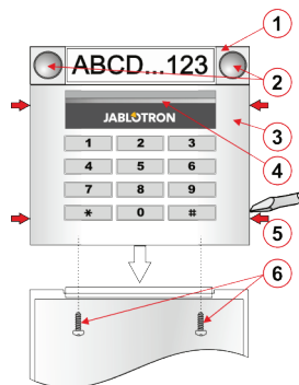
Obrázek 1: Popis vnějších a vnitřních částí výrobku
