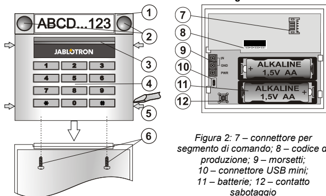
Figure 1: 1 – segmento di comando; 2 – pulsanti segmento; 3 – pulsante attivazione retroilluminato; 4 – modulo accesso con lettore RFID; 5 – schede per apertura modulo; 6 – viti copertura
