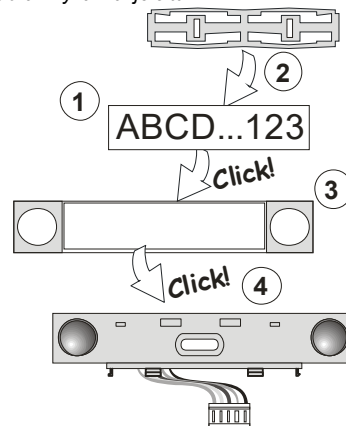
3. ábra: A címke behelyezése a vezérlő szegmensbe
