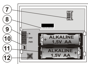
2. ábra: 7 – a vezérlő szegmens csatlakozója; 8 – gyártási sorozatszám; 9 – sorcsatlakozó; 10 – mini USB csatlakozó; 11 – elemek; 12 – szabotázskapcsoló
