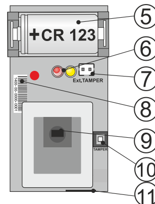
Rysunek 2.: 5 – uchwyt na baterię; 6 – diody LED; 7 – Gniazdo do podłączenia sabotażu z uchwytu JA-191PL; 8 – kod produkcji; 9 – sensor PIR; 10 – zatrzask obudowy; 11 – antena
