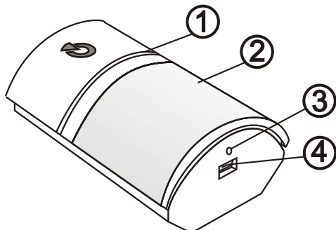
Rysunek 1.: 1 – diody LED; 2 – soczewka/optyka PIR; 3 – otwór na śrubę blokującą; 4 – zatrzask obudowy
