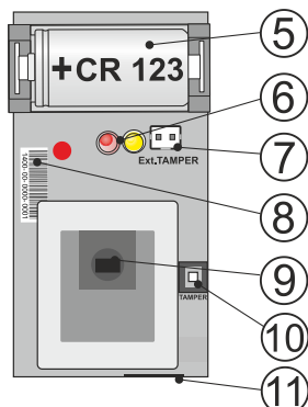
Figur 2: 5 – batteriholder, 6 – LED-indikatorer, 7 – JA-191PL eksterne sabotagestik, 8 – serienummer, 9 – PIR-sensor, 10 – dækslets sabotagekontakt, 11 – antenne
