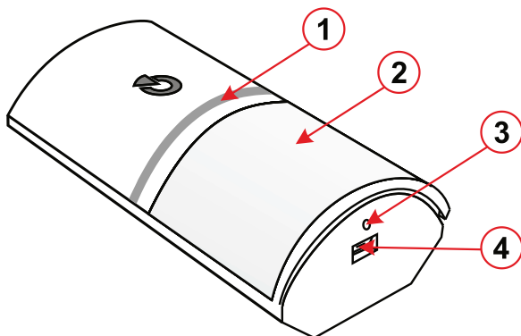
Obrázek 1.: 1 – světelné signálky; 2 – čočka PIR senzoru; 3 – otvor pro aretační šroubek; 4 – západka pro otevření/zavření
