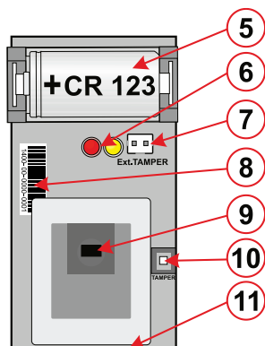
Obrázek 2.: 5 – pouzdro pro baterii; 6 – indikační signálky; 7 – konektor pro připojení sabotážního kontaktu držáku; 8 – sériové číslo; 9 – PIR senzor; 10 – sabotážní kontakt krytu; 11 – anténa
