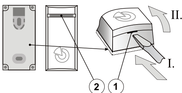
Figura: 1 – declanșator al butonului de apăsare al capacului; 2 – indicator de activare cu LED roșu
