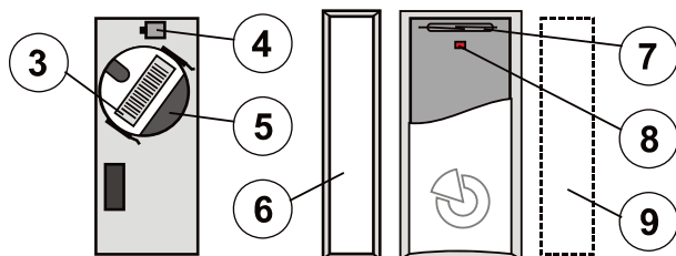
Figura: 3 – cod de producție; 4 – contact tamper; 5 – baterie; 6 – magnet permanent; 7 – senzor magnetic; 8 – indicator cu LED roșu pentru activarea detectorului; 9 – locație alternativă a magnetului permanent
