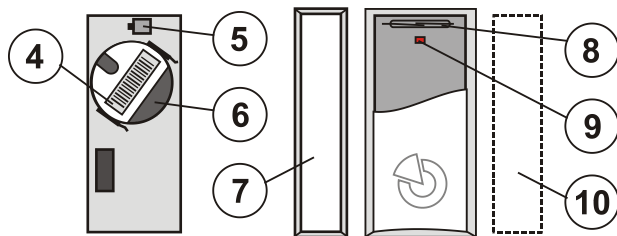
Bild: 4 – Seriennummer; 5 – Sabotageschalter; 6 – Batterie; 7 – Permanentmagnet; 8 – Magnetischer Sensor; 9 – rote Meldeleuchte der Melderaktivierung; 10 – alternative Anbringung des Permanentmagnets
