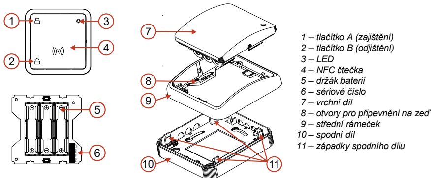
Obrázek 1: Popis vnějších a vnitřních částí výrobku
