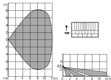
Obrázek 3.: Detekční charakteristika
