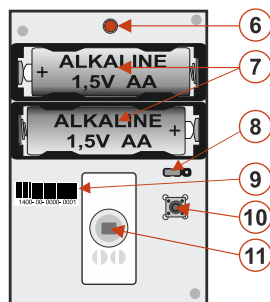
Obrázek 2.: 6 – LED indikátor; 7 – baterie; 8 – nastavovací propojka Imunity; 9 – sériové číslo; 10 – sabotážní spínač; 11 – PIR senzor
