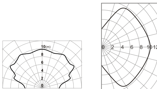
Obrázek: Detekční charakteristika detektoru GBS.
