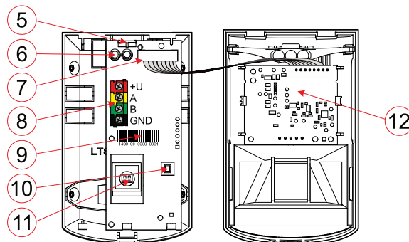
Figure 2 : Description des parties internes du produit
