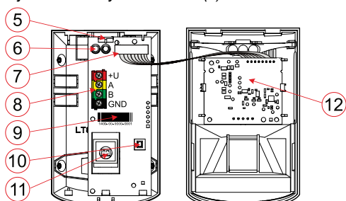
Obrázek 2: Popis vnitřních částí výrobku
