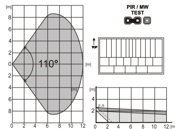
obrázek 2.: Charakteristiku pokrytí lze změnit použitím alternativní čočky:
