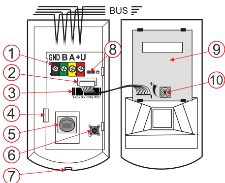
obrázek 1: 1 – svorkovnice sběrnice; 2 – konektor mikrovlny; 3 – sériové číslo; 4 – západka aretace DPS; 5 – PIR senzor; 6 – sabotážní spínač; 7 – západka krytu; 8 – testovací propojka; 9 – MW senzor; 10 – nastavení citlivosti MW
