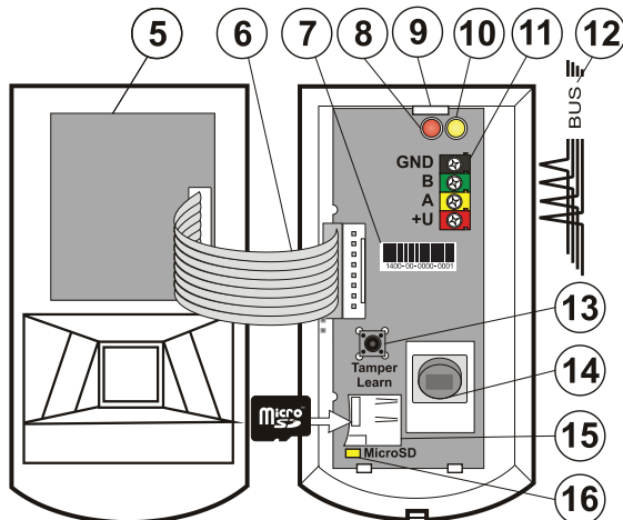
Рисунок: 5 – Модуль камеры; 6 – соединительный кабель; 7 – код изделия; 8 – красный светодиодный индикатор; 9 – язычок печатной платы; 10 – желтый светодиодный индикатор; 11 – клеммы шины; 12 – магистральная шина; 13 – тамперный контакт; 14 – пассивный инфракрасный датчик; 15 – карта памяти Micro SD; 16 – желтый индикатор карты памяти Micro SD
