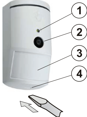
Рисунок: 1 – вспышка для освещения; 2 – линза камеры; 3 – линза пассивного инфракрасного детектора; 4 – язычок крышки;
