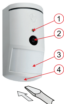
Obrázek: 1 – fotoblesk pro přisvětlení; 2 – objektiv kamery; 3 – čočka PIR detektoru; 4 – západka krytu
