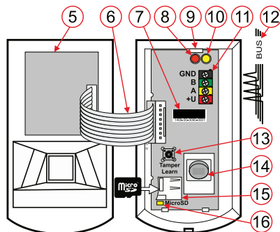
Obrázek: 5 – modul kamery; 6 – propojovací kabel; 7 – sériové číslo; 8 – červená LED; 9 – západka desky elektroniky; 10 – žlutá LED; 11 – svorkovnice sběrnice; 12 – kabel sběrnice; 13 – sabotážní spínač; 14 – PIR senzor; 15 – paměťová karta micro SD; 16 – žlutá LED micro SD karty.
