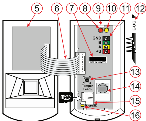
Obrázek: 5 – modul kamery; 6 – propojovací kabel; 7 – sériové číslo; 8 – červená LED; 9 – západka; 10 – žlutá LED; 11 – svorkovnice sběrnice; 12 – kabel sběrnice; 13 – sabotážní spínač; 14 – PIR senzor; 15 – paměťová karta Micro SD; 16 – žlutá LED micro SD karty.
