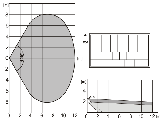
Figura: Característica de detección del detector PIR
