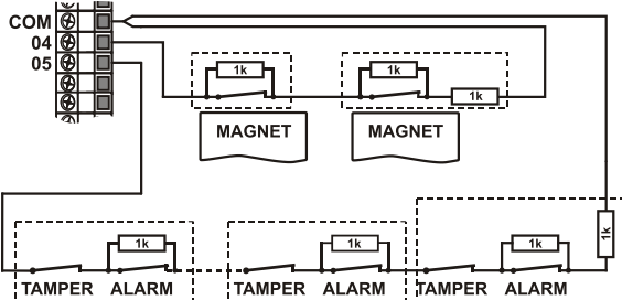
Obrázek: Příklad zapojení více periférií na jeden vstup smyčkou dvojitě vyvažovanou odporem 1k. Zapojení svorek 4-COM: Magnetický detektor s poplachovým výstupem. Zapojení svorek 5-COM: Detektory s poplachovým výstupem a s ochranným kontaktem krytu.
