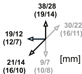
Afbeelding 3: Oriëntatiedetectieafstand - activatie / deactivatie aan een niet-magnetisch (magnetisch) oppervlak
