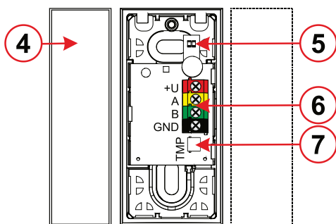
Figuur 2: Beschrijving van de interne onderdelen van de detector: 4 - permanente magneet; 5 - LED-indicatoren; 6 - busklemmen; 7 - sabotageschakelaar.
