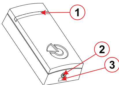
Figuur 1: Beschrijving van het externe deel van de detector: 1 - LED lichtgeleider; 2 - borgschroef; 3 - dekselvergrendeling
