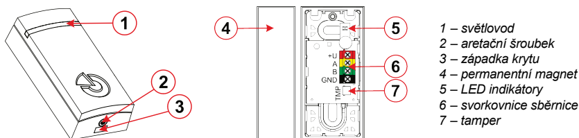
Obrázek 1: Popis vnějších a vnitřních částí výrobku
