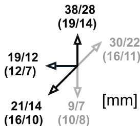
3. ábra: Orientációérzékelési távolság - bekapcsolás / kikapcsolás bekapcsolva nem mágneses (mágneses) felületen
