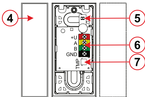
2. ábra: Az érzékelő belső részeinek leírása: 4 - állandó mágnes; 5 - LED kijelző; 6 - buszcsatlakozók; 7 - szobatózás kapcsoló.
