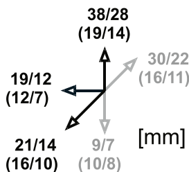
Figure 3 : Distance de détection de l'orientation - activation / désactivation sur une surface non magnétique (magnétique)
